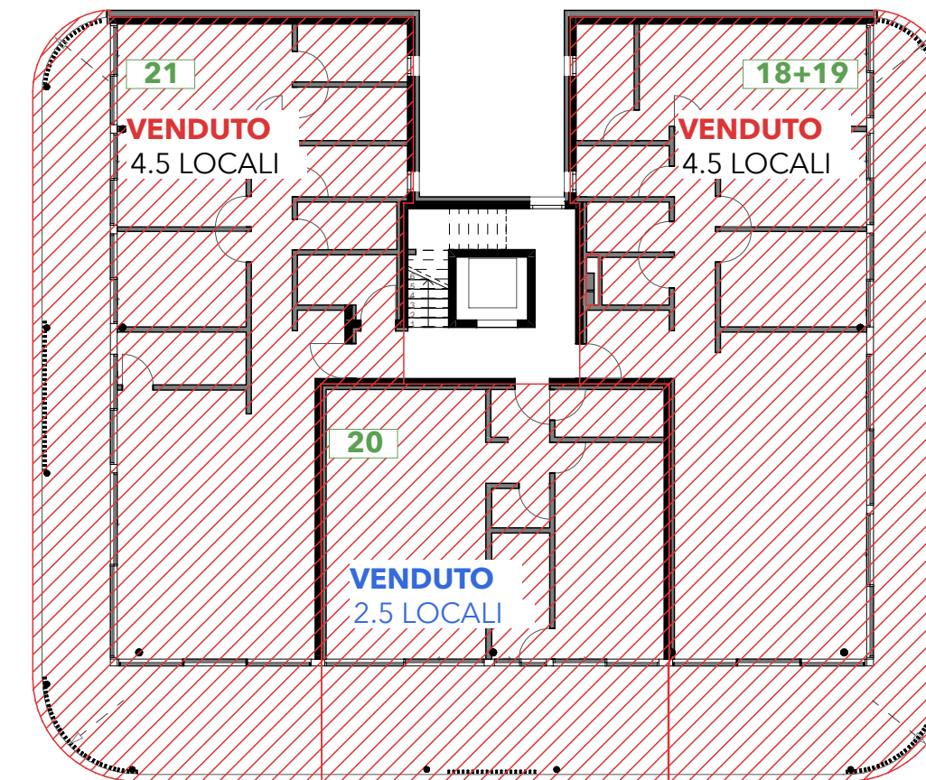
LIVELLO +5. SCALA 1:200
