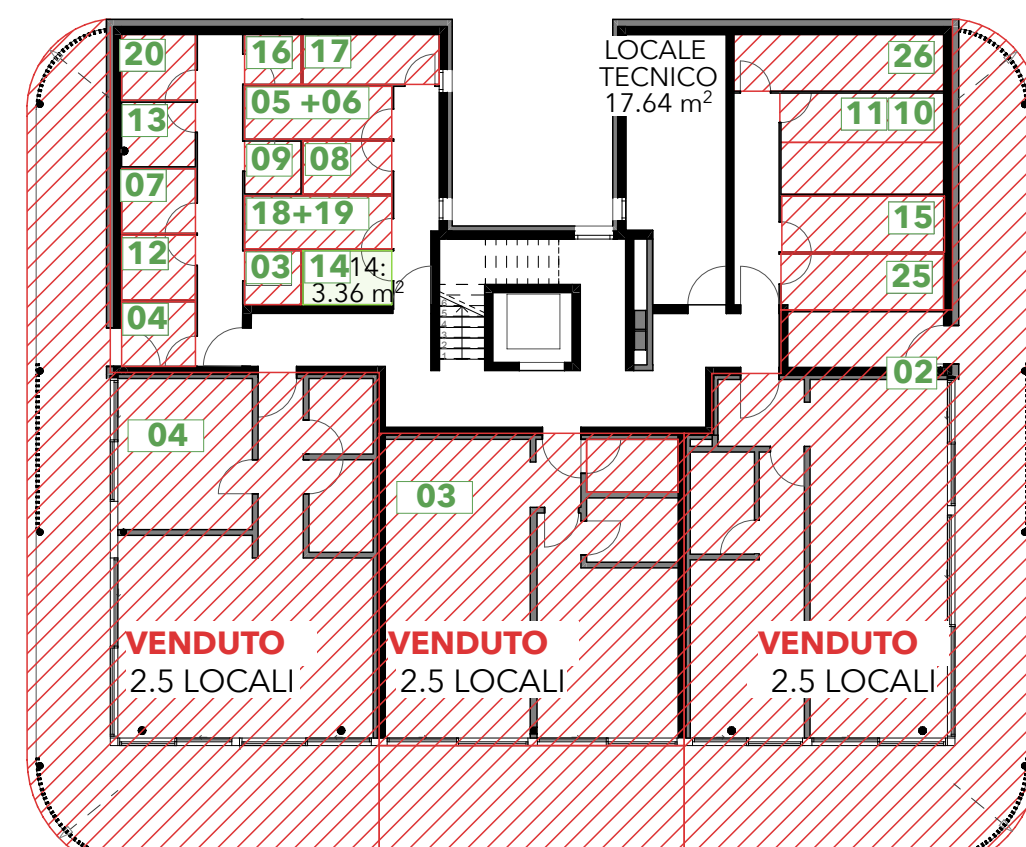
LIVELLO +1. SCALA 1:200
